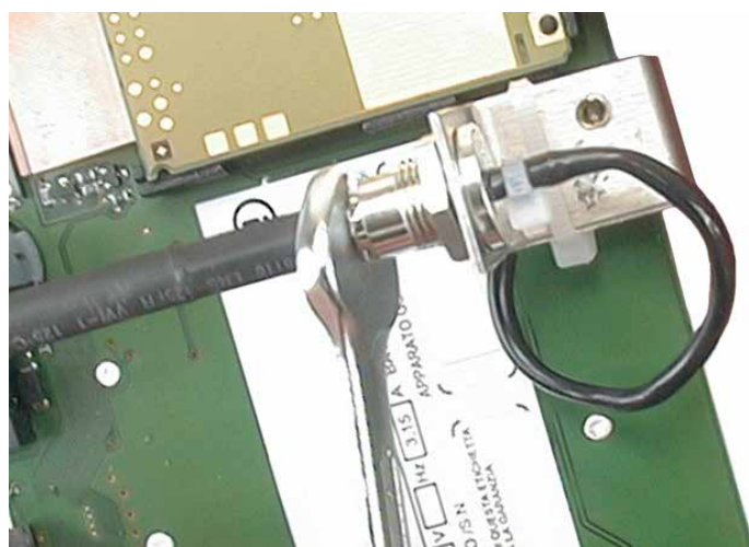
Serraggio del connettore FME (ADANTTRH)
